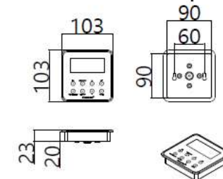
TOLO Steuerdisplay
